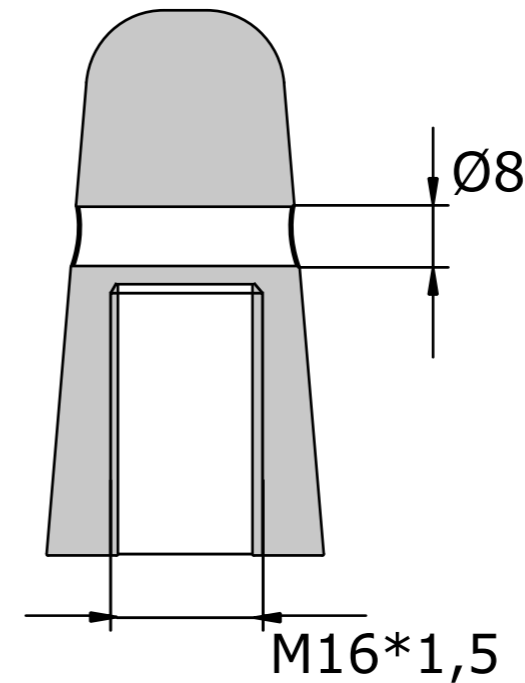
Schnittansicht A-A
